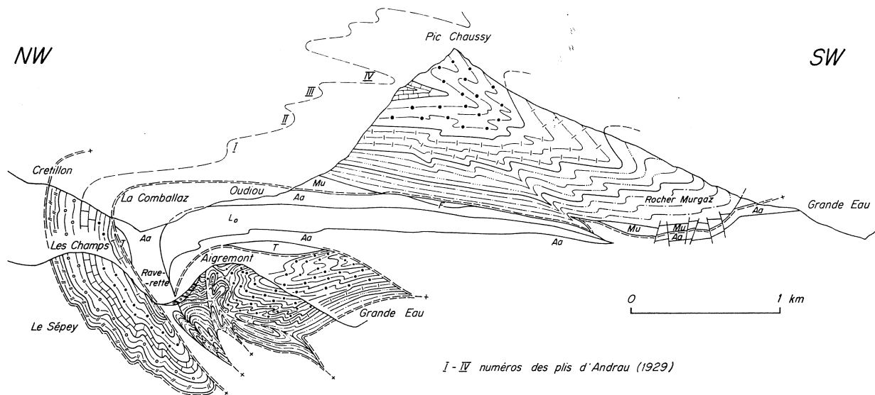
Fig. 1: Profil à travers l'extrémité SW de la nappe du Niesen et son soubassement (Légende: voir planche I; T = Trias, L 0 = Lias de l'écaille d'Oudiou, Mu = Trias et Lias de l'écaille de Murgaz, Aa = Aalénien, F = Flysch ultrahelvétique).
